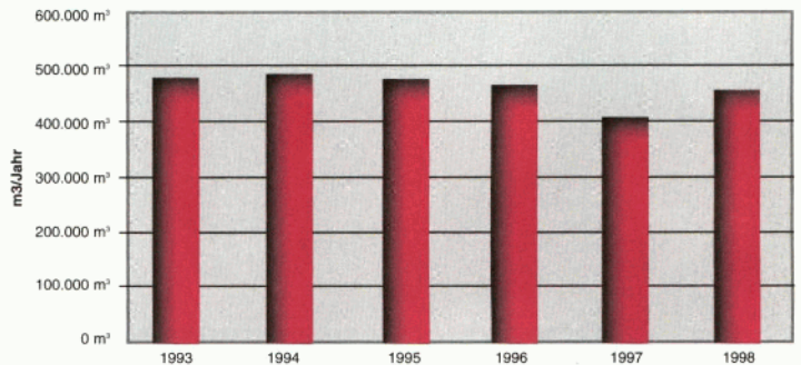
Wasserverbrauch der Stadtgemeinde Liezen
