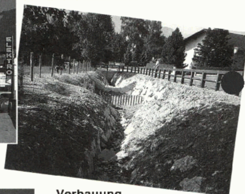
Verbauung des Grützengrabens zur weiteren Baulanderschließung östlich der Tausingsiedlung
