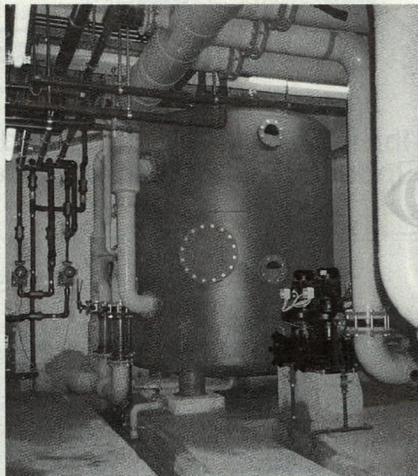
Neue Filteranlage mit Kessel und Pumpe zur Reinigung des Badewassers.
