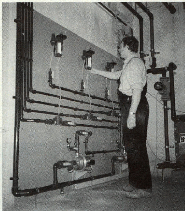
Chlordosierungsanlage, in welcher der Chlor- gehalt des Wassers gesteuert wird.
